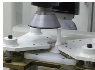
図2 専用加工機による脚部の研削作業
